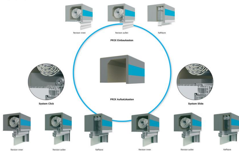
PRIX Baukasten: Die Neue Generation Rolladenkästen
